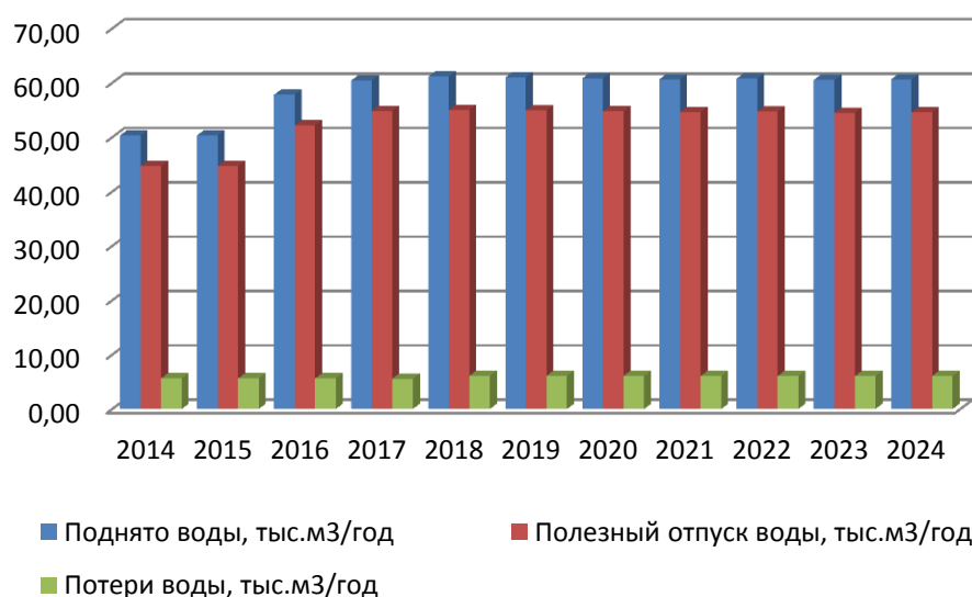
Рисунок 3-8. Перспективный водный баланс Сосновского сельского поселения (годовой)
