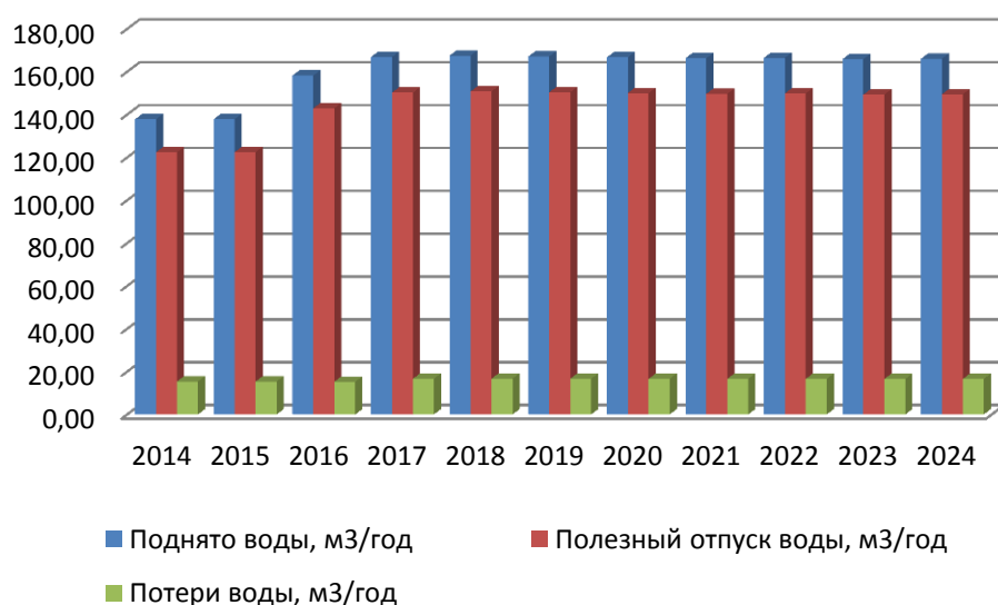
Рисунок 3-9. Перспективный водный баланс Сосновского сельского поселения (среднесуточный)
